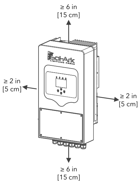
Figura 2: Espacios mínimos de unidad
