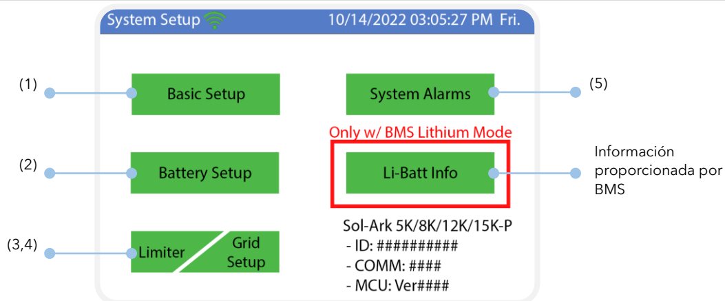
Figura 24: Pantalla de configuraciones
