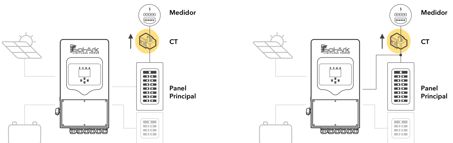
Figura 15: Instalación de CTs para a) interruptor de retroalimentación y b) derivación de línea
